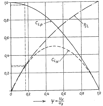
Bild 5 (links). Drucksprung im Gebläse. Daten des gestrichelt eingezeichneten Beispiels: u_s = 30 \text{ m/s} ; u_v = 5 \text{ m/s} ; \Psi = 0,167 ; \Delta p_{VE} / (\rho/2 \cdot u_s^2) = 0,97
