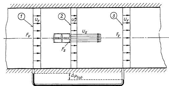
Bild 2. Prinzipskizze des Lüftungsabschnittes mit Strahlgebläse
