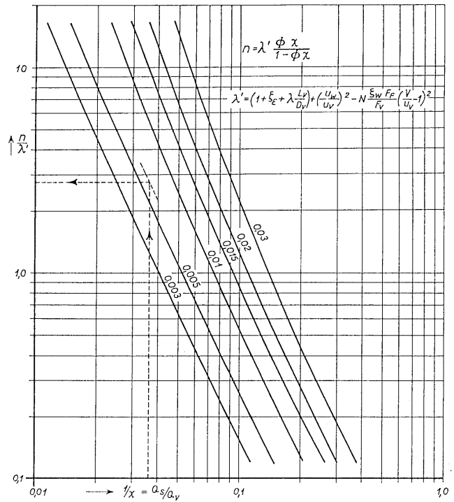
Bild 8. Kurven zur Bestimmung der Anzahl Strahlventilatoren.
